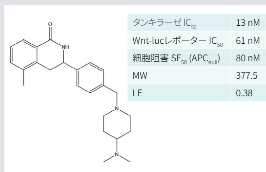
図1:Domainexで設計および合成されたイソナフトキノントンキラーゼ阻害物質の例
